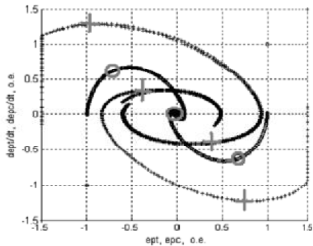
Рис 3. Результат кластерного анализа выходного сигнала нечеткого регулятора тока и скорости от ошибки и скорости ошибки на входах
