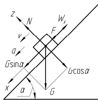
Рис. 6. Розрахункова схема руху потягу в режимі гальмування
