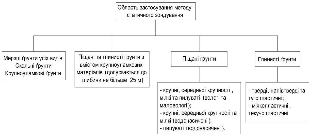
Рис. 1. Схема застосування методу статичного зондування
