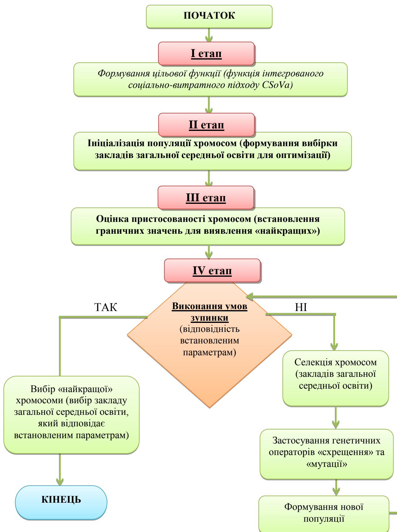
Рис.3.1. Блок-схема генетичного алгоритму для оптимізації територіальної організації закладів загальної середньої освіти
