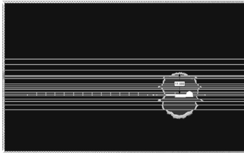
Рис. 2. Качественная картина зоны разрушения выработанного пространства при R_{\text{лсв}} \text{ песчаника} = 10 \text{ МПа} (отходе лавы от разрезной печи на 10 м)
