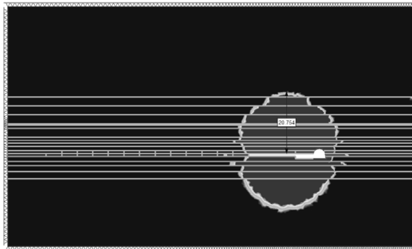
Рис. 3. Качественная картина зоны разрушения выработанного пространства при R_{\text{лсв}} \text{ песчаника} = 15 \text{ МПа} (отходе лавы от разрезной печи на 15 м)
