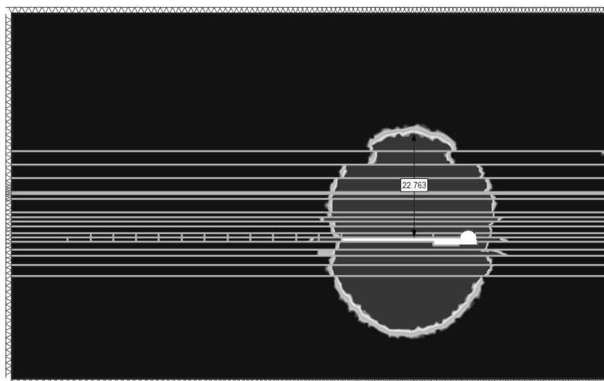
Рис. 3. Качественная картина зоны разрушения выработанного пространства при R_{\text{лсв}} \text{ песчаника} = 15 \text{ МПа} (отходе лавы от разрезной печи на 15 м)
