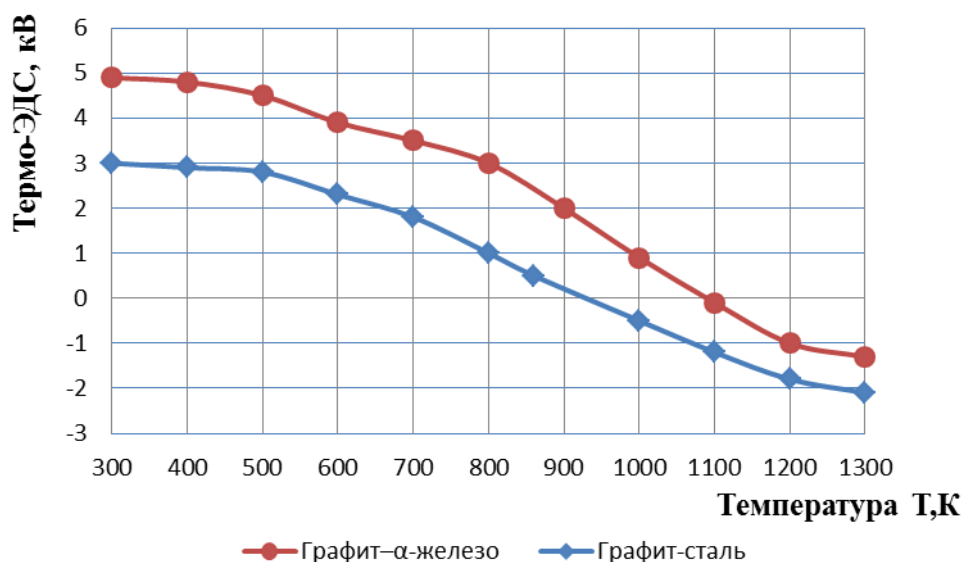
Рис. 3. Характер изменения контактной разности потенциалов на границе материалов: 1 – графит-α-железо; 2 – графит-сталь
