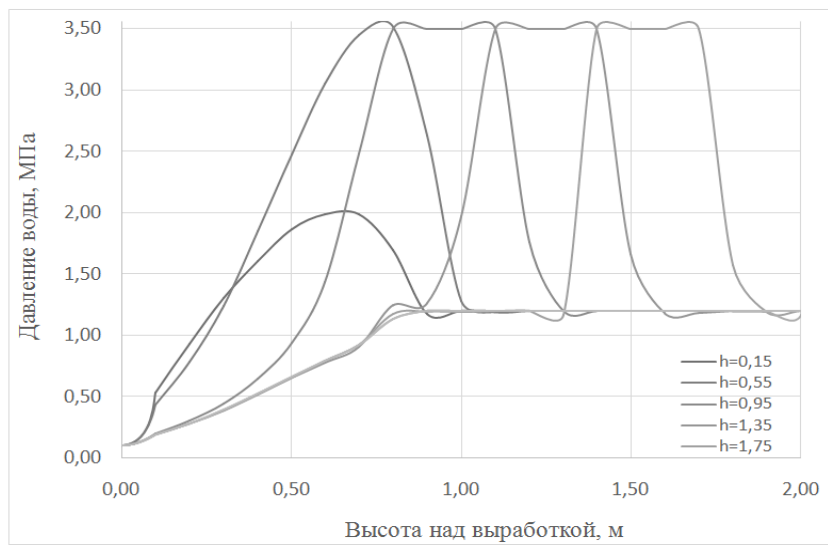
Рис. 7. Изменение давления воды в зависимости от высоты расположения подрабатываемого пропластка
