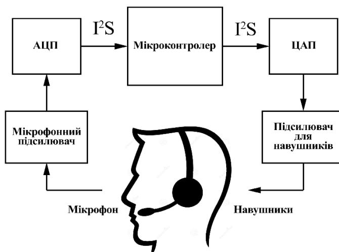
Рис. 1. Структурна схема пристрою
