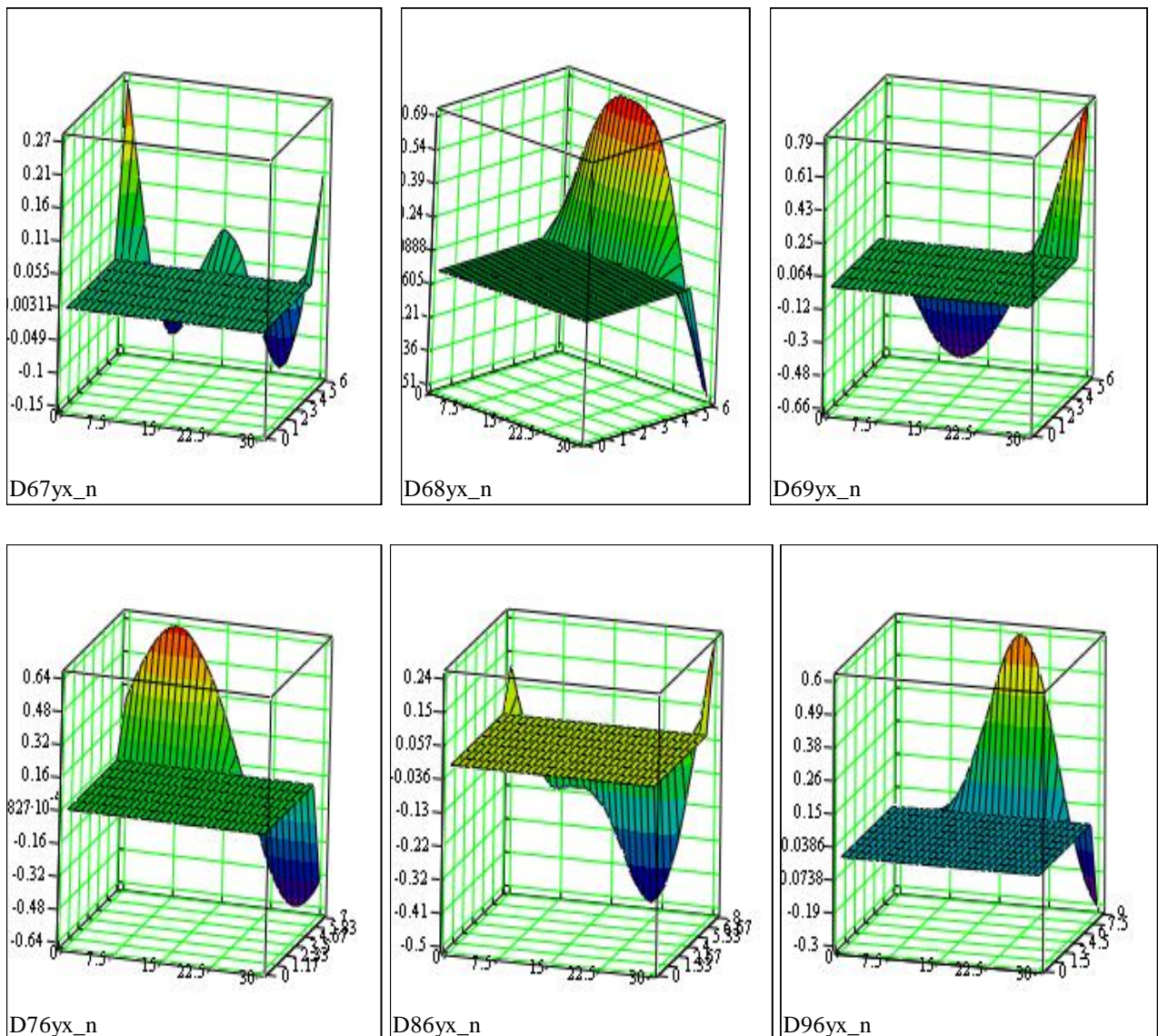
Рис. 1. Нормированные взаимодисперсионные функции экспериментальных реализаций мгновенных значений потребляемой мощности привода барабанной мельницы ММС 70*23 между заполнением \varphi = 47\% (1) и всеми технологически возможными остальными
