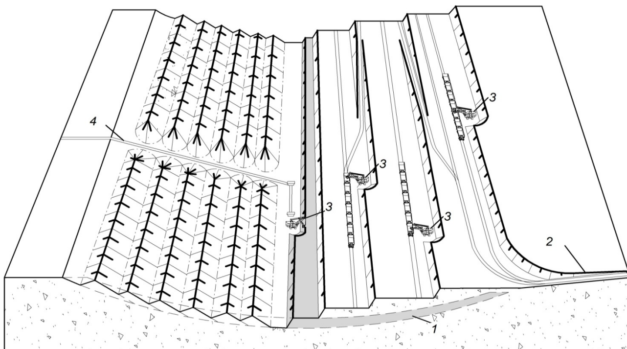
Рисунок 1.1 – Комбінація траншейного способу розкриття родовища з безтраншейним:
