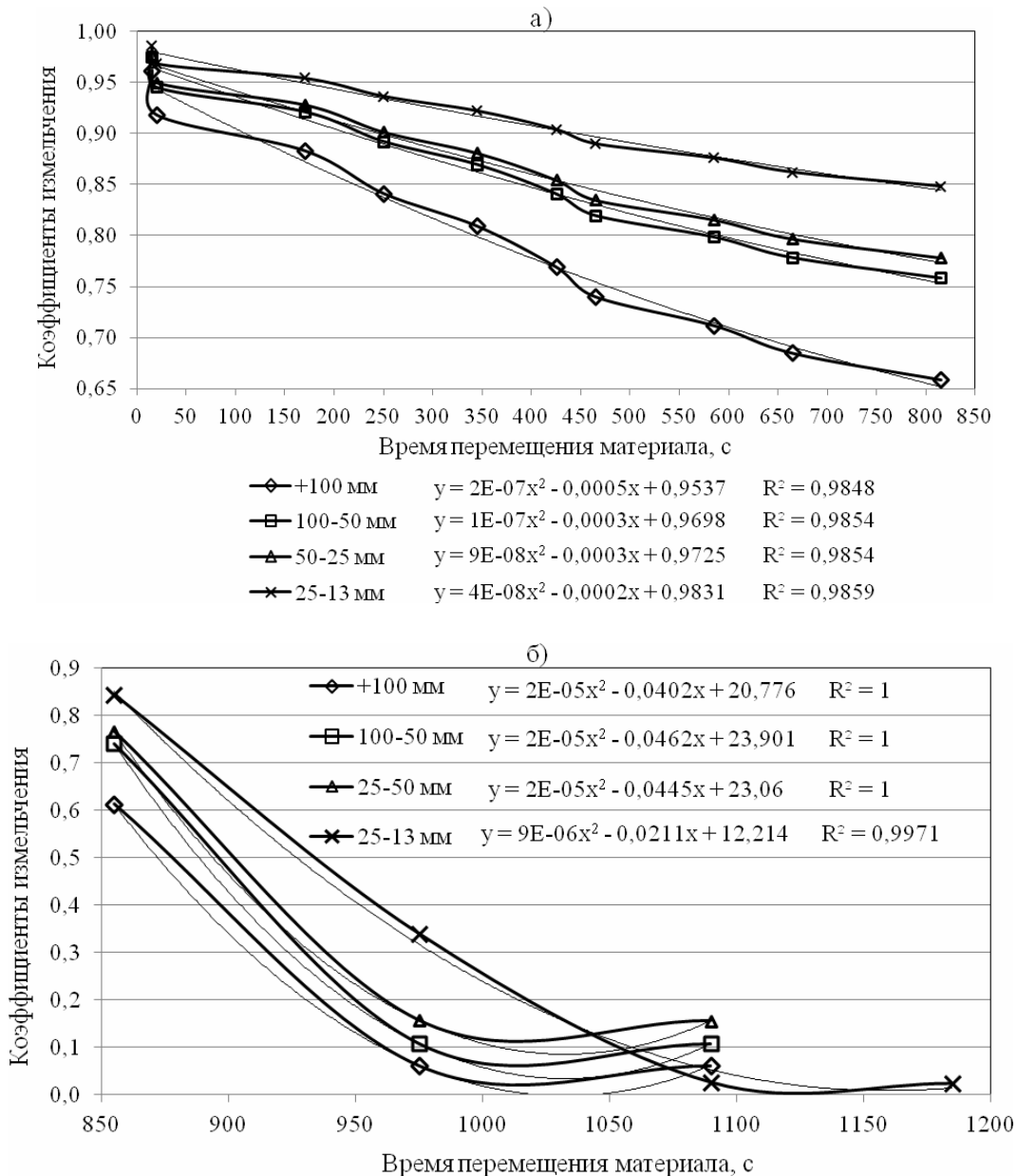
Рис. 1. Кривые изменения коэффициентов измельчения крупных классов во времени: а) в отделении углеприема и углеподготовки; б) в отделении обогащения
