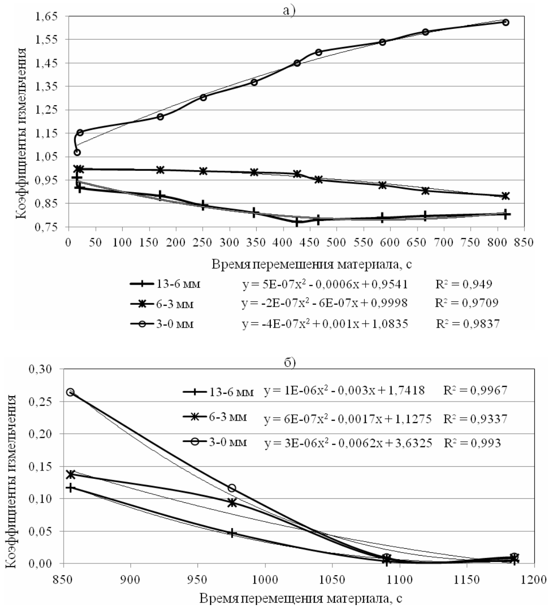
Рис. 2. Кривые изменения коэффициентов измельчения мелких классов во времени: а) в отделении углеприема и углеподготовки; б) в отделении обогащения
