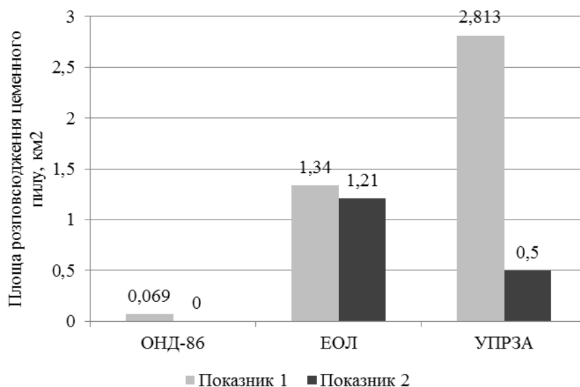
Рис. 4. Площі впливу цементного пилю на навколишнє середовище і населення району
