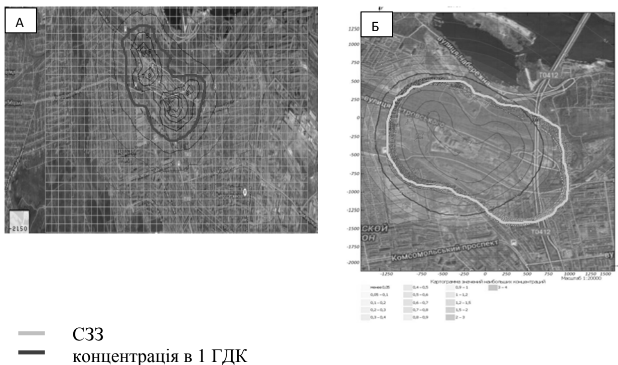
Рис. 3. Карта розсіювання цементного пилу А) оригінальне зображення за «ЕОЛ+» накладене на космоснімок місцевості; Б) карта розсіювання цементного пилу (УПРЗА «Еколог»)
