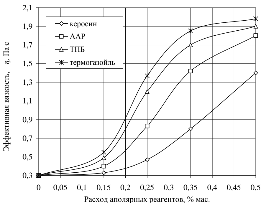
Рис. 2. Зависимость эффективной вязкости от расхода реагентов
