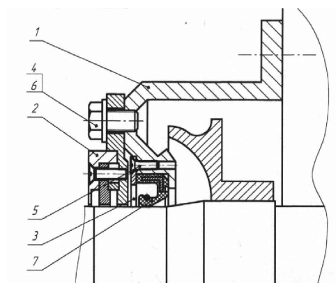
Рис. 4. Герметизатор компрессора
