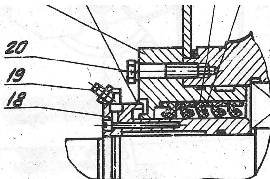
Рис. 7. Штатное уплотнение барабана
