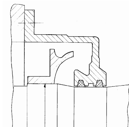
Рис. 3. Штатное уплотнение
