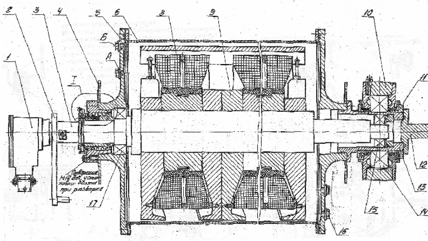
Рис. 8. Барабан электромагнитный
