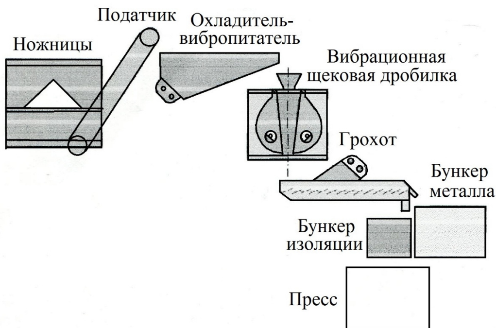
Рисунок 2 – Схема криогенной технологии для переработки кабельных отходов (НГУ)
