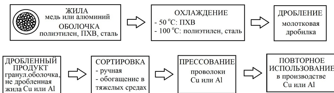
Рисунок 1 – Схема криогенной линии для переработки кабельных отходов (Франция)
