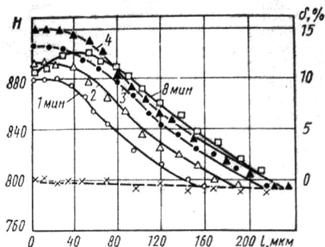
Рис. 1. Распределение микротвердости H по толщине цементованного слоя ( l – расстояние от поверхности) стали 12Х2Н4А и степень его упрочнения \delta при разном времени обдувки дробью (цифры у кривых).
