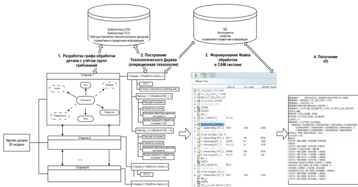
Рис.2. – Модель процесса формирования управляющей программы на оборудование с ЧПУ в ИТС
