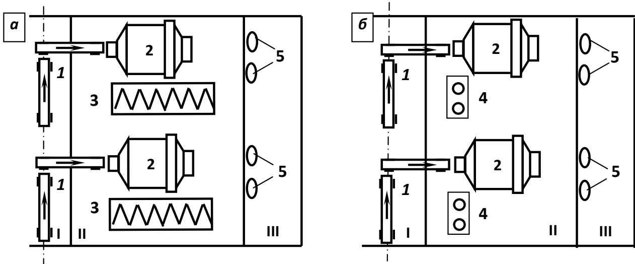
Рис. 1. Схема однорядного компонування млинів у секціях при одностадійному подрібненні:
