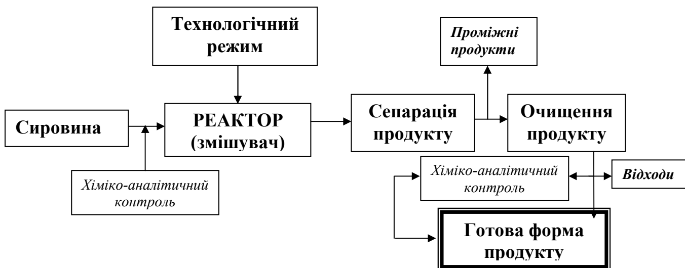
Рис. 1. Блок-схема типового технологічного процесу хімічного виробництва
