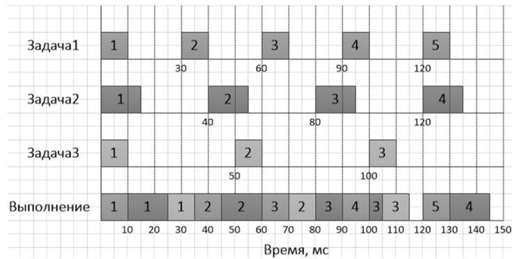
Рисунок 3 – Пример работы алгоритма LLF
