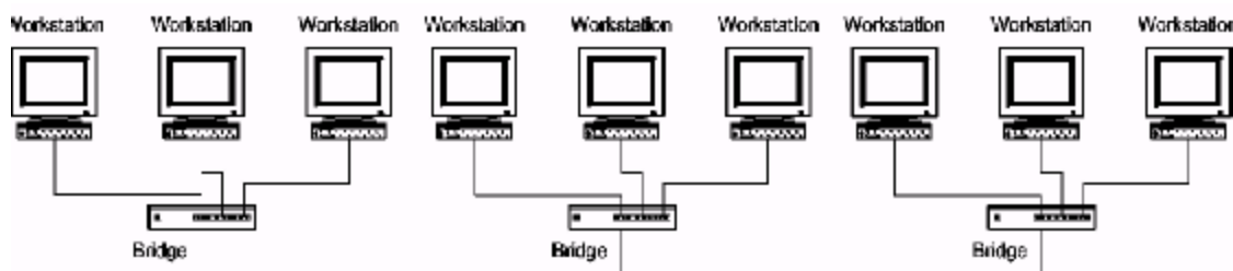
Рис. 8.4. Локальна мережа з топологією "зірка-шина"
