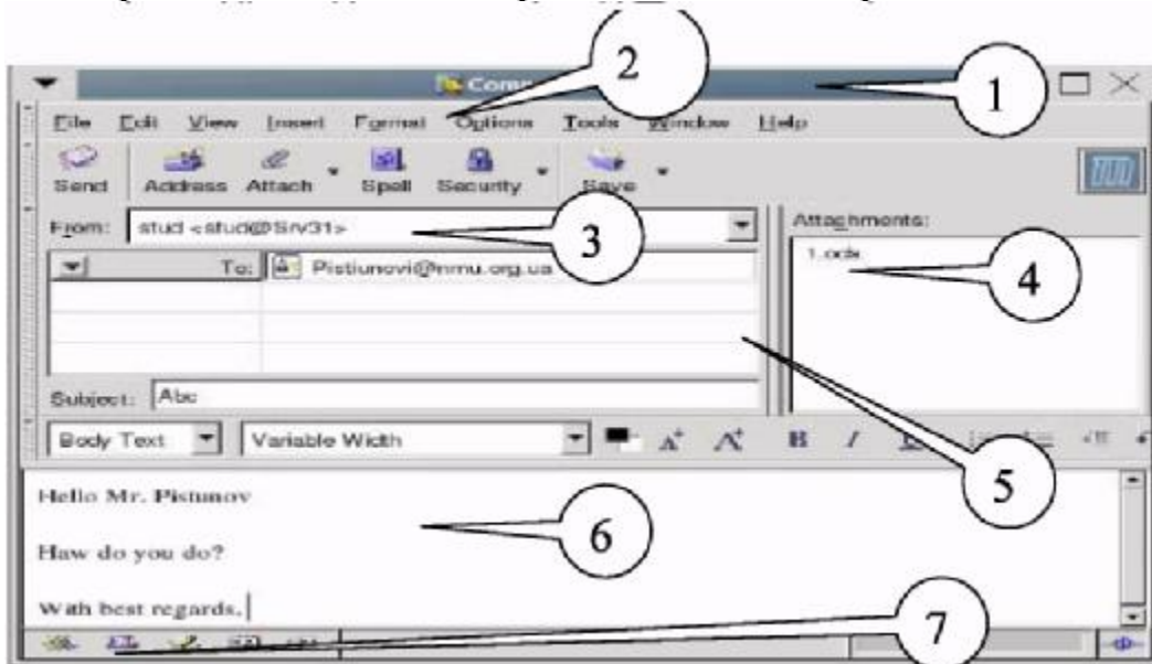
Рис. 9.10. Вікно для створення поштових повідомлень мейлера Mozilla
