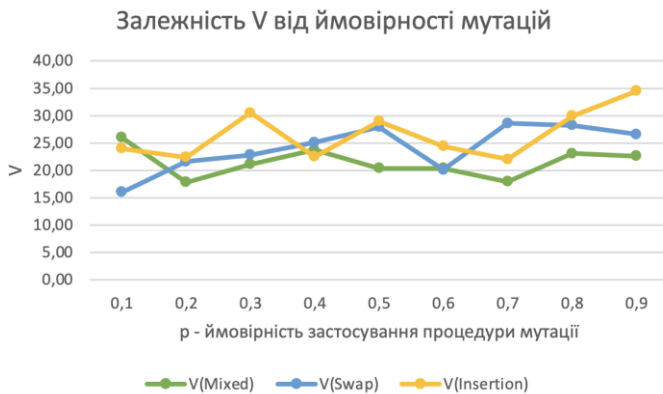
Рисунок 1 – Графіки залежності V від ймовірності мутації обміном, вставками та змішаної мутації
