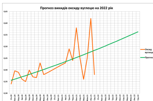
Рисунок 1 – Графік прогнозу викидів оксиду вуглецю
