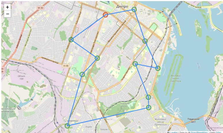
Рисунок 2 – Результат побудови маршруту алгоритмом GRASP
