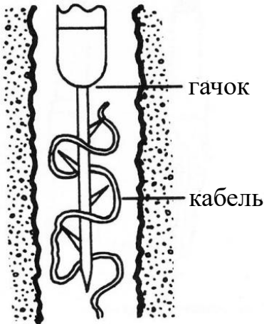
Рис. 1. – Схема роботи гачка з обмежувачем
