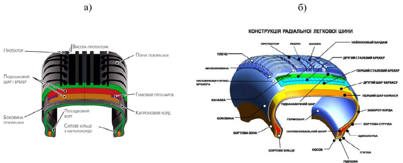
Рис. 1 Будова автошини [1]
