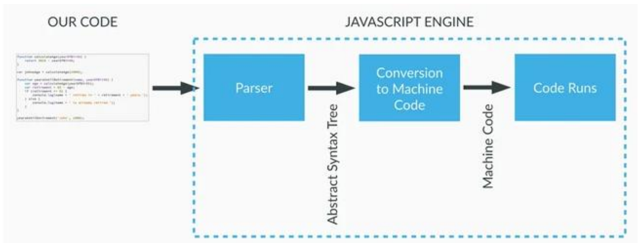
Рис.2.1 Схема роботи JavaScript [17]
