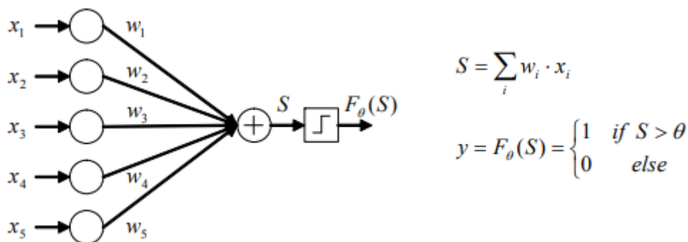
Рис.2.2 Одношаровий персептрон з п'ятьма булевими входами та одним виходом
