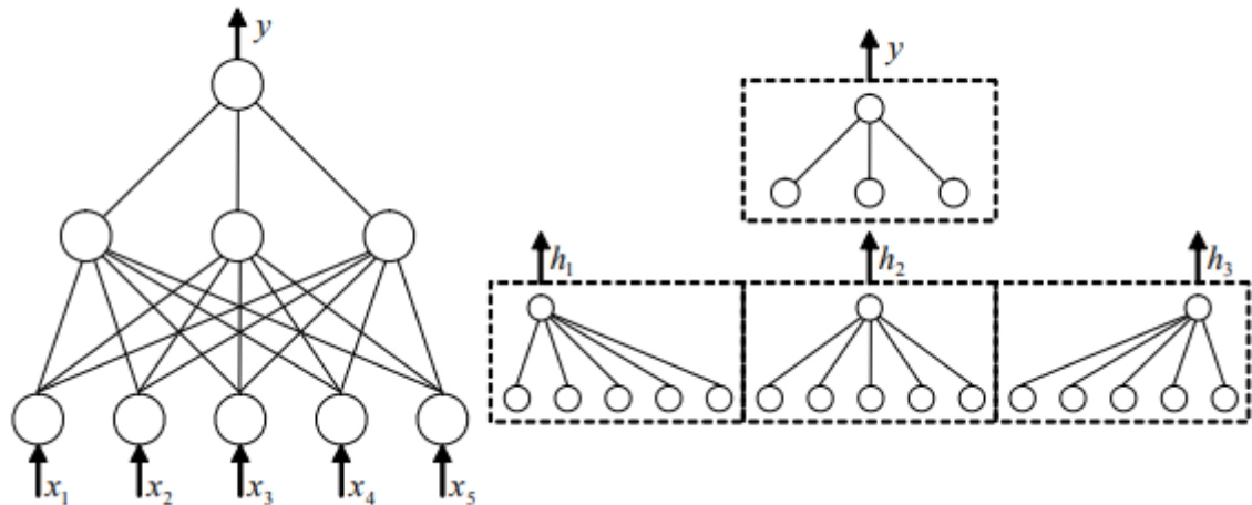
Рис.2.3 Локальний підхід до вилучення правил
