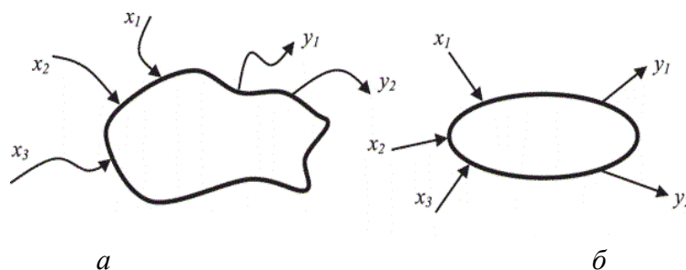
Рисунок 3.3 – Схема побудови моделі: а – досліджувана система, б – модель
