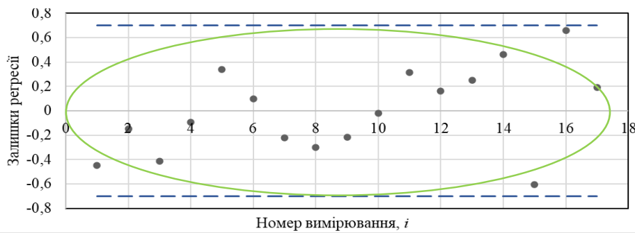
Рисунок 6.3 – Графік розподілу залишків регресії (пунктиром показано інтервал (2S_\varepsilon; -2S_\varepsilon) нормального розподілу залишків регресії)
