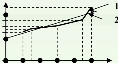
Рисунок 4.9 – Лінії регресії: 1 – експериментальна, 2 – вибіркочеву
