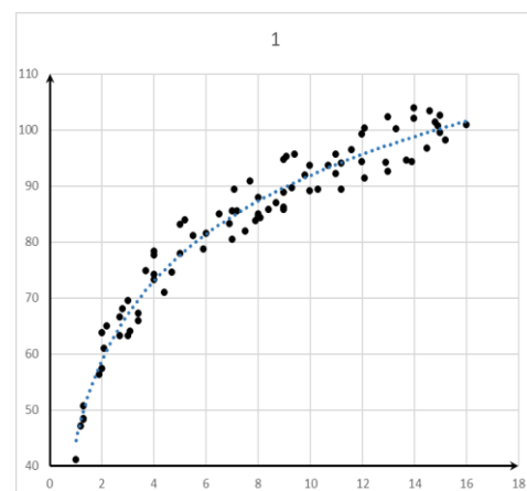
Рисунок 4.7 – Параболічна залежність Рисунок 4.8 – Логарифмічна залежність
