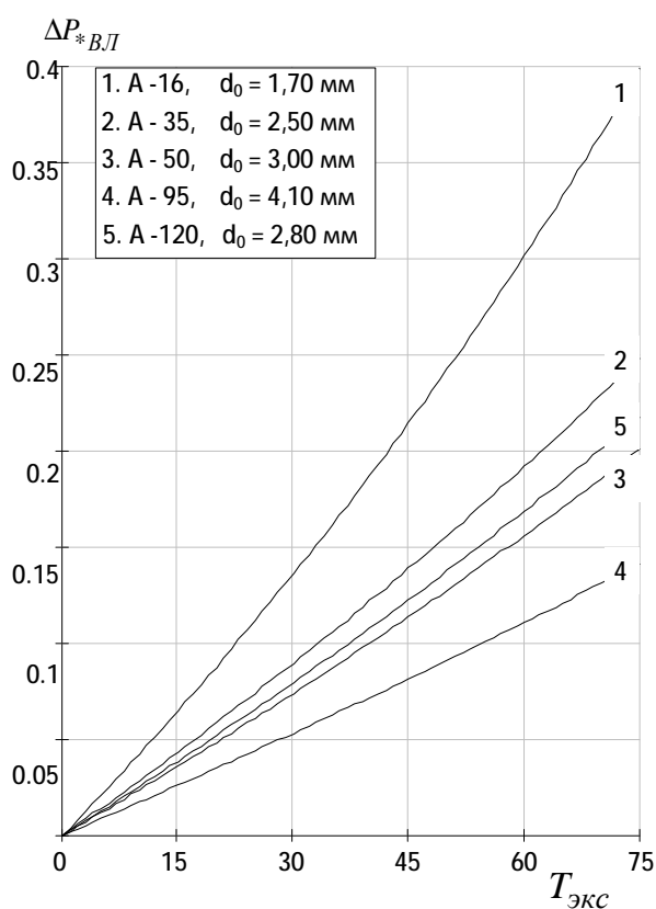
Рис.3. Характер изменения нагрузочных потерь в воздушных ЛЭП в процессе эксплуатации для Dd_0 = 1,75 мкм/г
