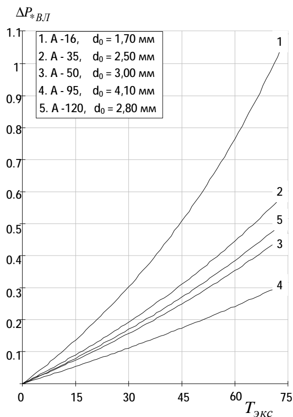
Рис.2. Характер изменения нагрузочных потерь в воздушных ЛЭП в процессе эксплуатации для Dd_0 = 3,5 мкм/г
