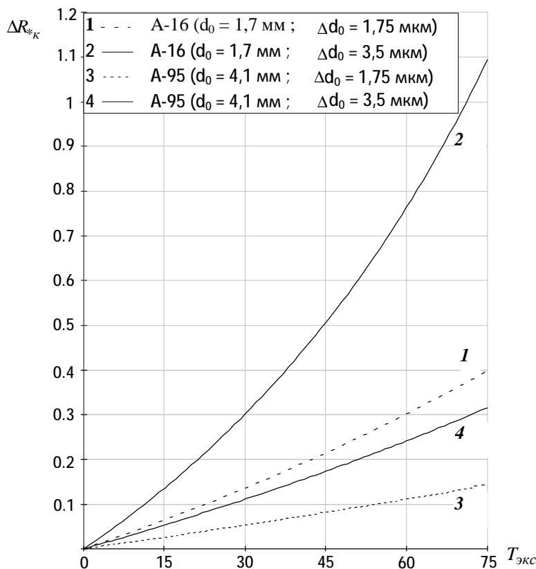
Рис.1. Зависимость \Delta R_{*к} = f(T_{экс}, \Delta d_0) для проводов марки А-16 и А-95 при крайних значениях скорости коррозии
