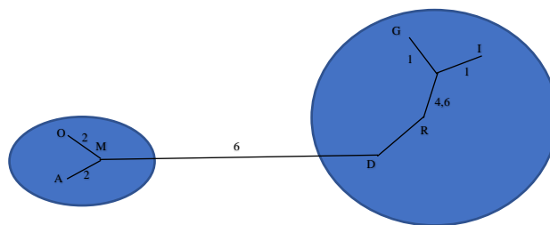
Рис. 1.17 – Алгоритм мінімального дерева, що покриває
