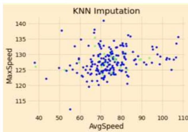
Рис. 1.9 - Метод k-найближчих сусідів
