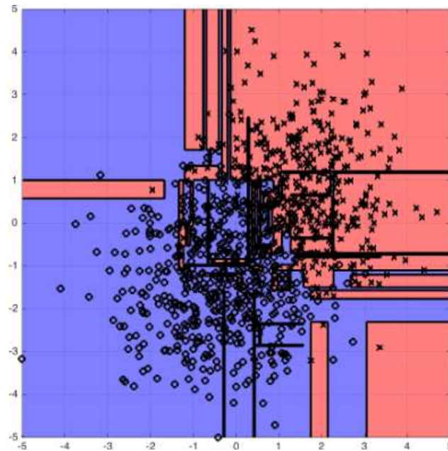
Рис. 15 – перенавчання дерева
