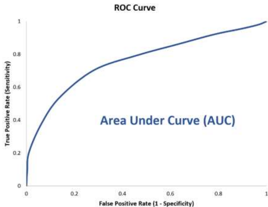
Рис. 1.12 – ROC-крива
