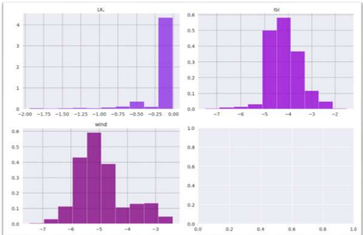
Рис. 2.9 – Гістограми після трансформації
