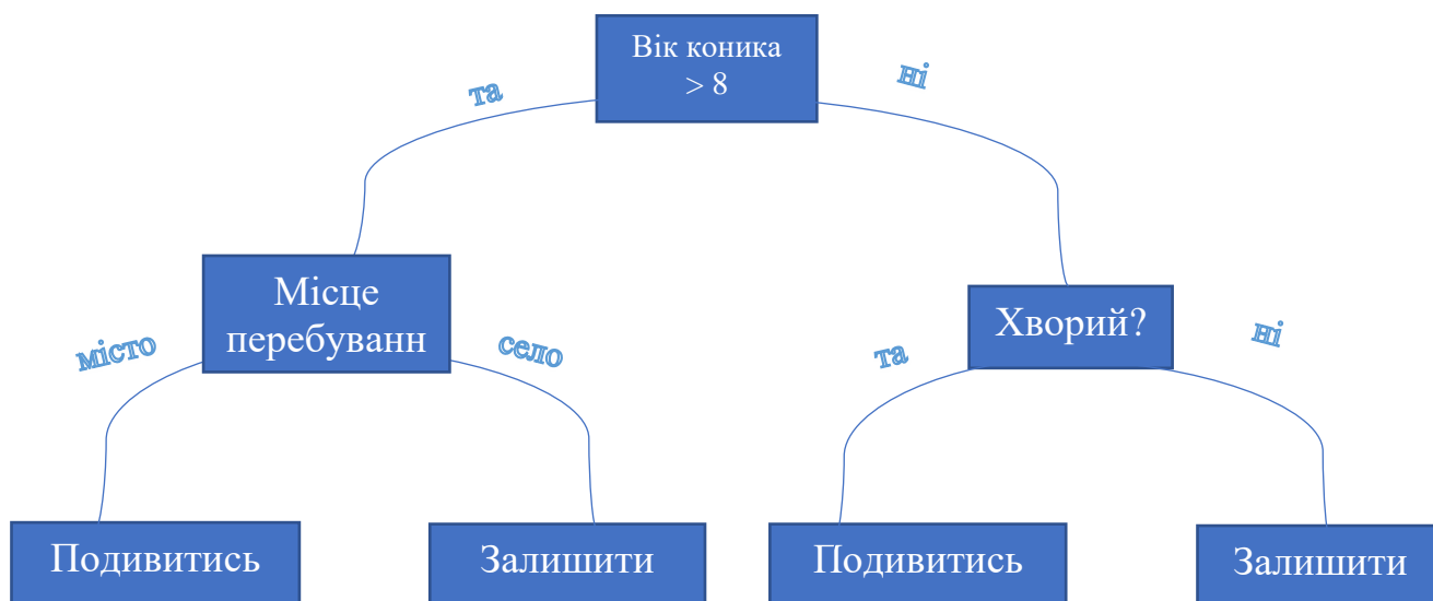
Рис. 1.14 – Древо рішень
