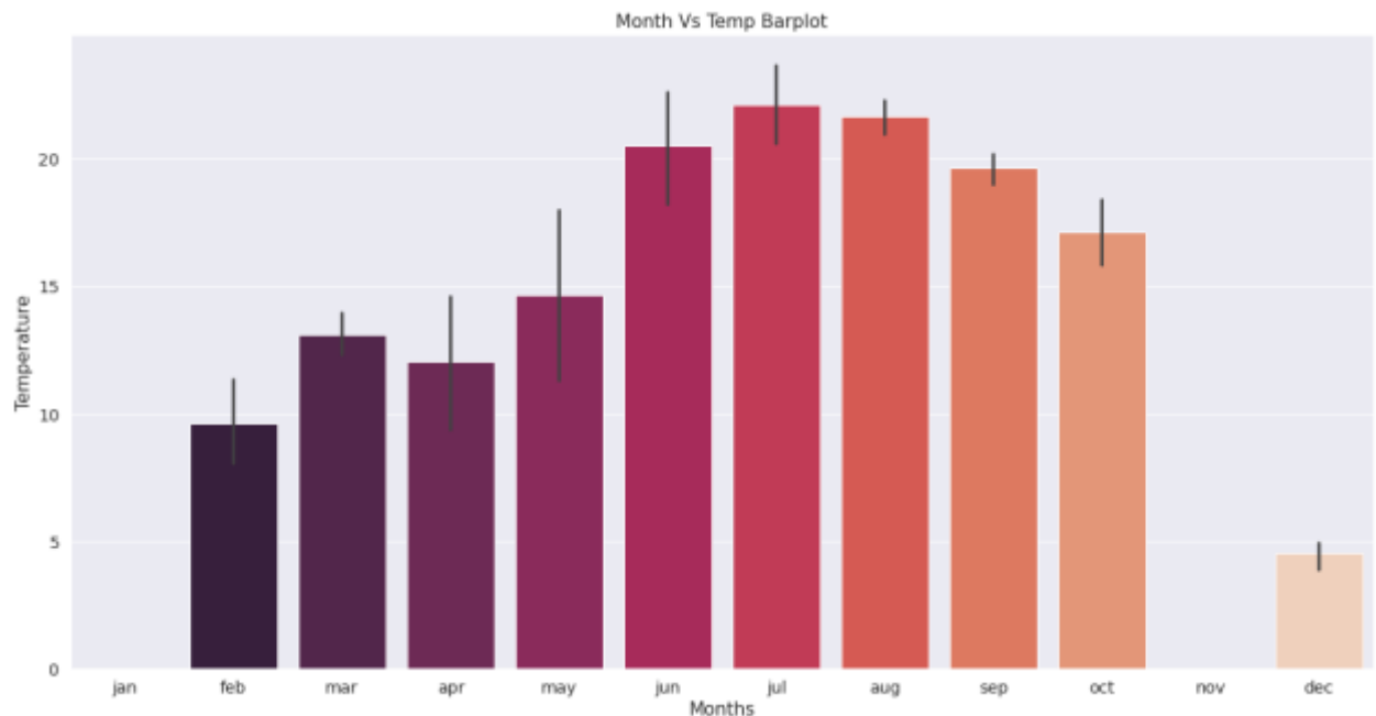
Рис. 2.2 – Температура повітря за місяцями
