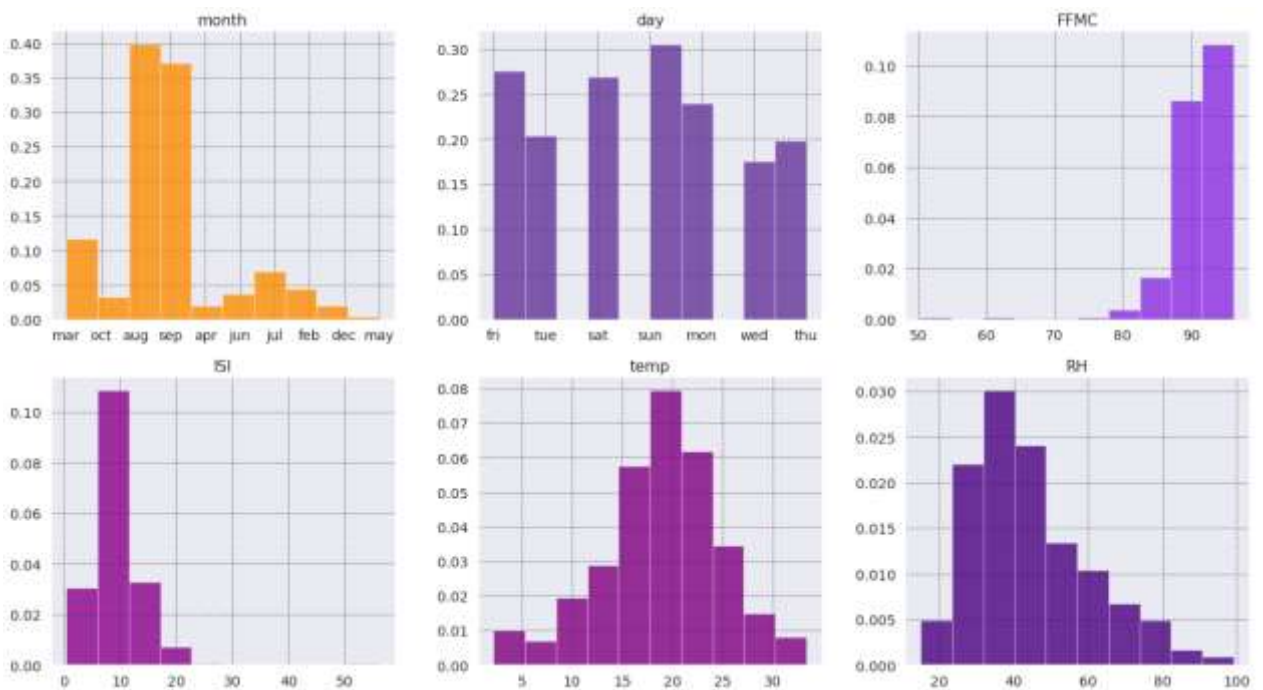
Рис. 2.4 – Гістограми основних ознак
