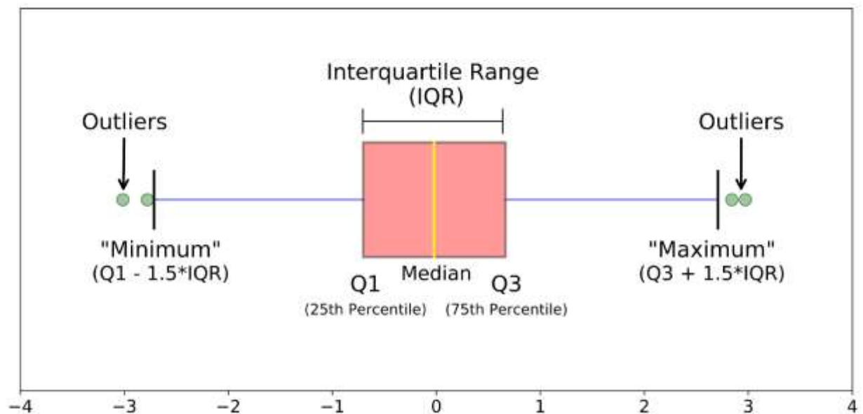
Рис. 1.4 – Коробчата діаграма
