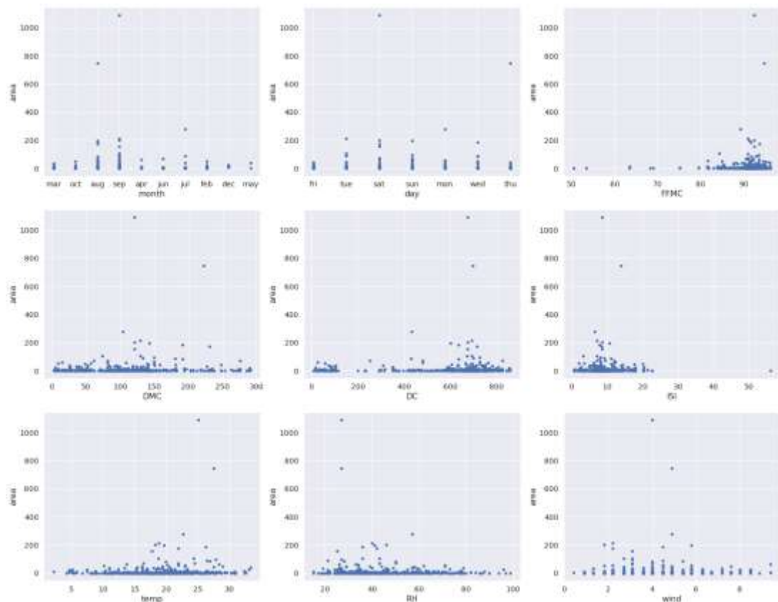
Рис. 2.3 - Огляд даних про наявність лінійного зв'язку з цільовою ознакою
