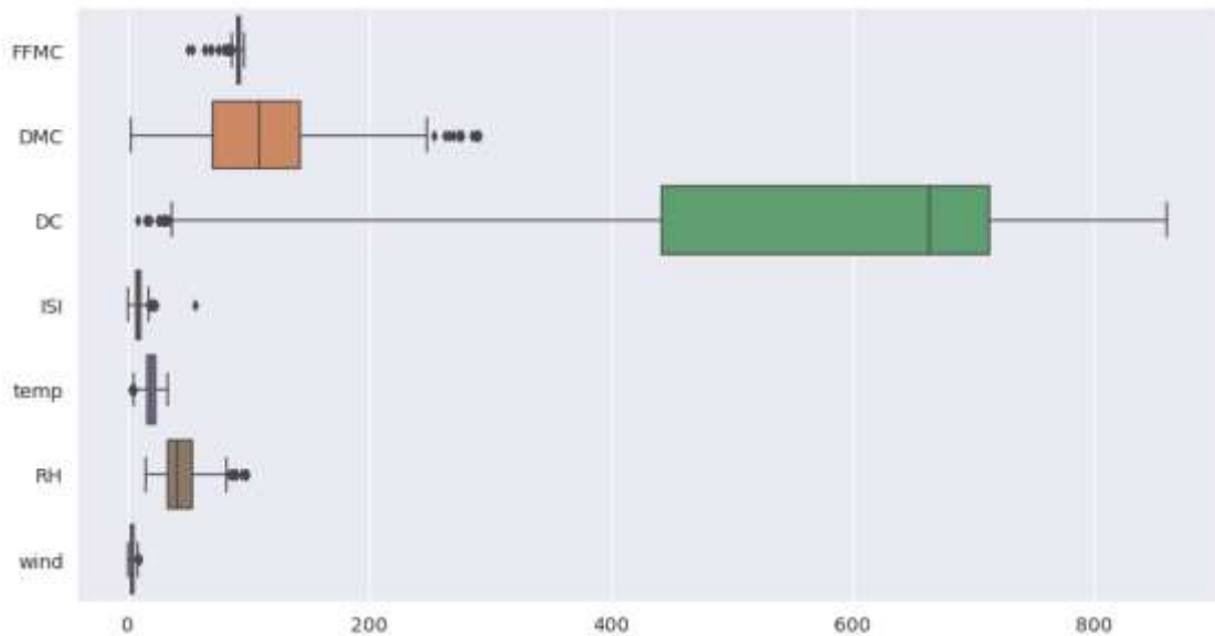
Рис. 2.6 – Коробчасті діаграми
