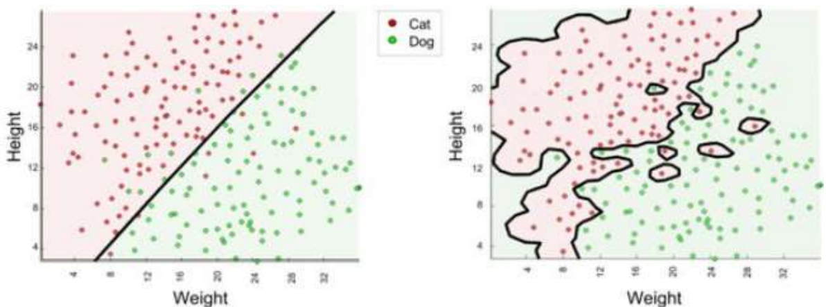
Рис. 1.16 – порівняння адекватної моделі з перенавченою
