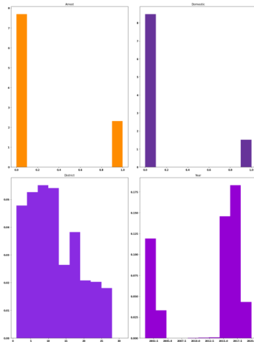
Рис. 2.13 – Графік розподілу ознак
