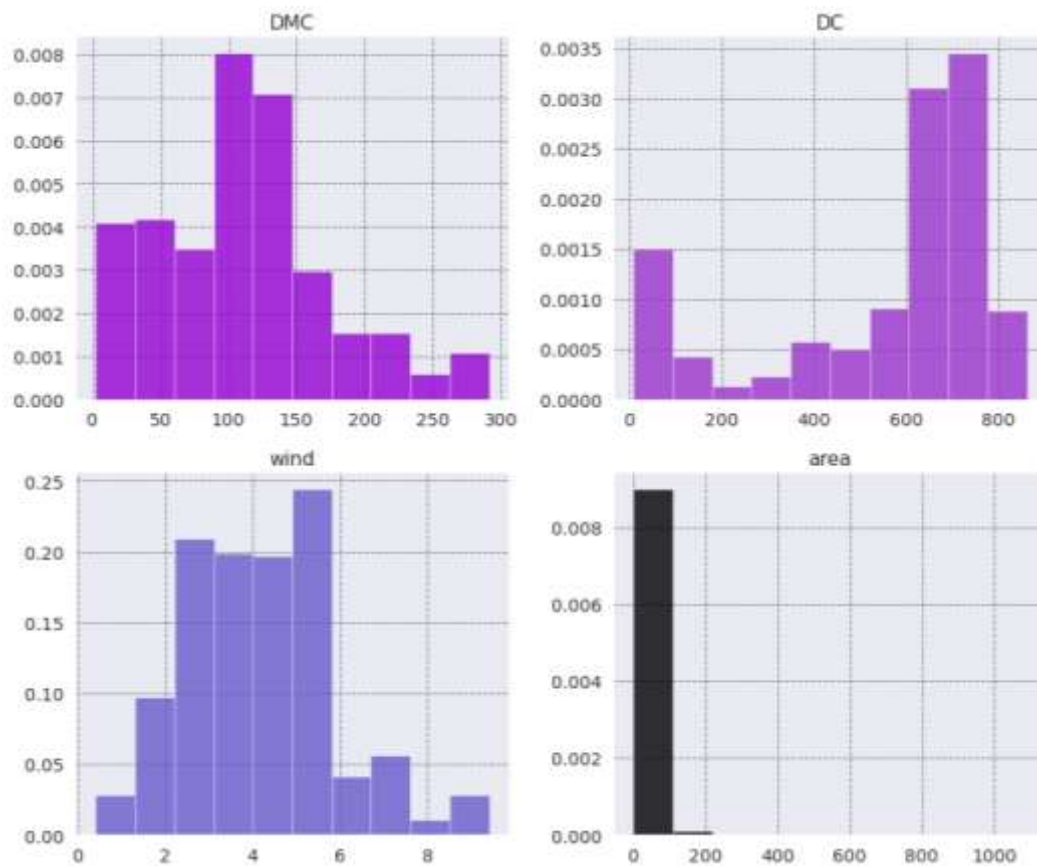
Рис. 2.5 – Гістограми основних ознак
