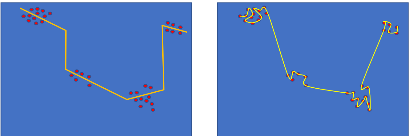
Рис. 18 – Порівняння бустингів.
