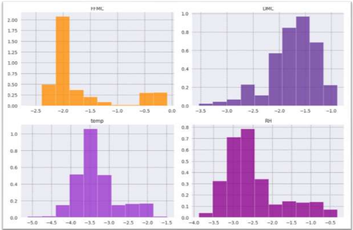
Рис. 2.8 – Гістограми після трансформації
