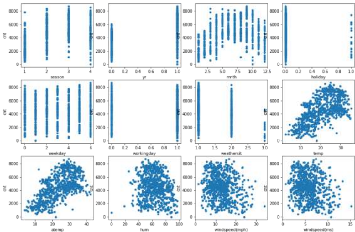
Рис. 1.1 – графіки залежності факторів відносно цільового значення
