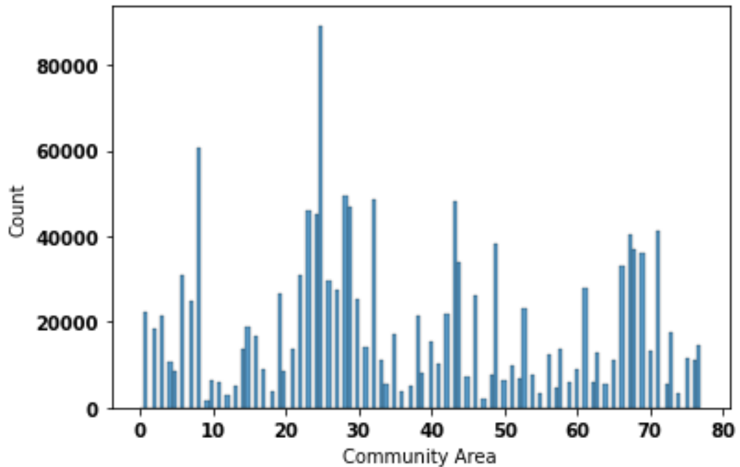
Рис. 2.14 – Графік кримінальності за районами
