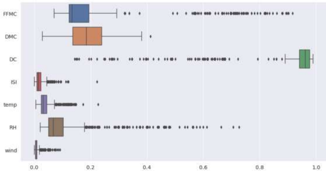
Рис. 2.7 – Коробчасті діаграми після трансформації
