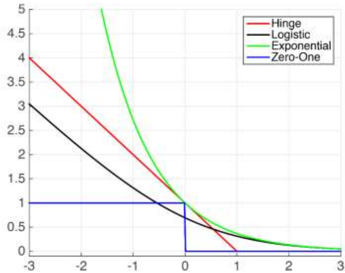
Рис. 1.11 – Функція втрат
