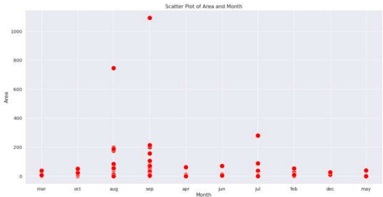
Рис. 2.1 – Площа займання за кожним місяцем, кількість займань
