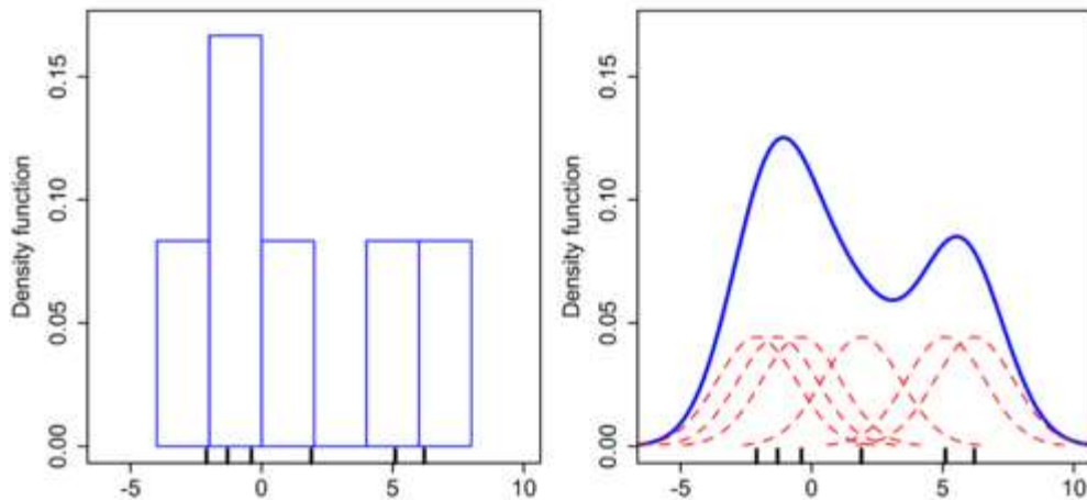
Рис. 1.3 – Ядерна оцінка щільності та гістограма
