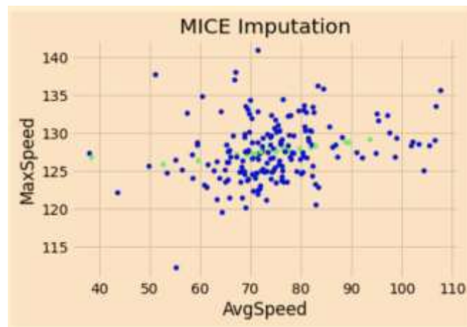
Рис. 1.10 – Заповнення пропусків за допомогою MICE
