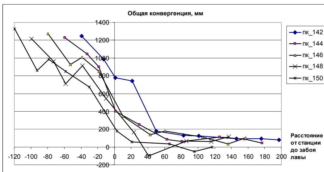
Рис. 2 - Сводный график общей конвергенции 159-го сборного штрека
