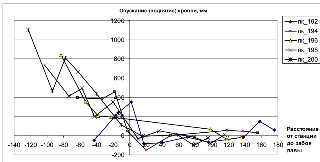
Рис. 6 - Сводный график опускания (поднятия) кровли 163-го сборного штрека
