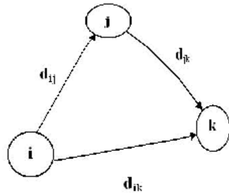
Рис. 2. Треугольный оператор
