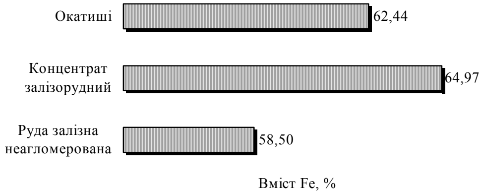
Рис. 3. Якісна характеристика продукції залізорудних гірничо-збагачувальних комбінатів
